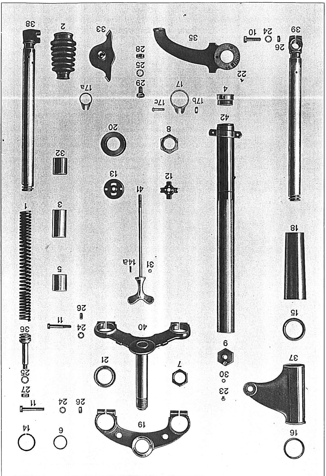
Vorderradgabel, Federung
